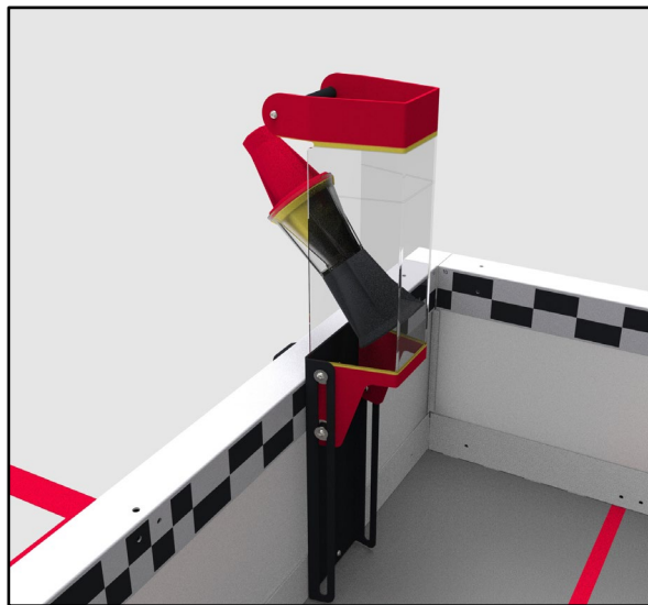
图 SG11-2: 当导入桶抬提起后，得分物可以从导入桶顶部背部导入
