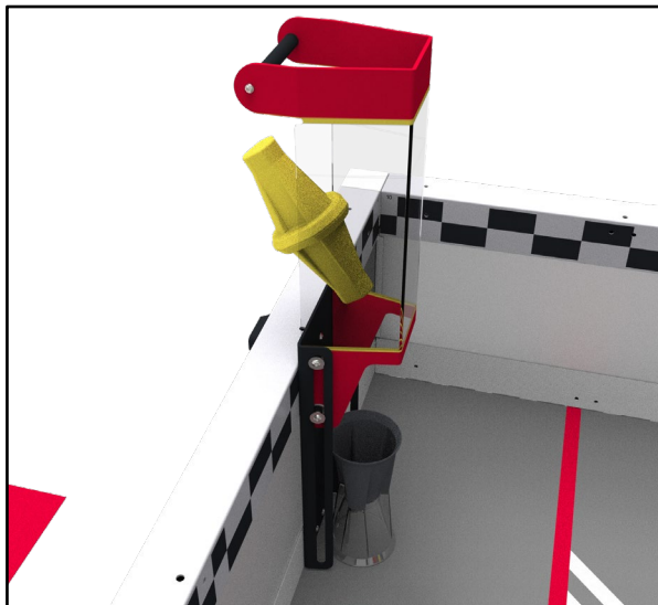
图 SG11-2: 当导入桶抬起后，得分物可以从导入桶顶部背部导入
