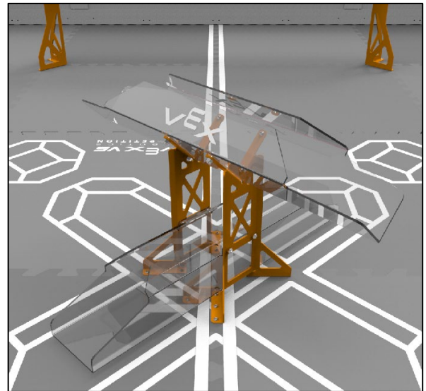
图 G-2: 一个中央得分桥
